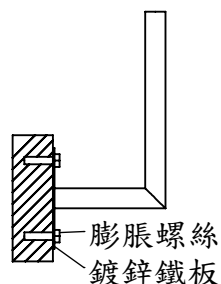
(一)挖孔灌漿埋設式 (二)底座式 (三)夾具固定式 (四)彎曲附壁式
