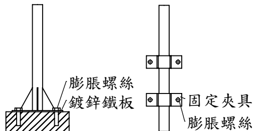
(一)挖孔灌漿埋設式 (二)底座式 (三)夾具固定式 (四)彎曲附壁式
